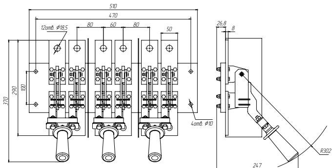
Рис. 9 Габаритные и установочные размеры разъединителя типа РЕ19-44/45/46-31170 с рукояткой для полюсного оперирования
